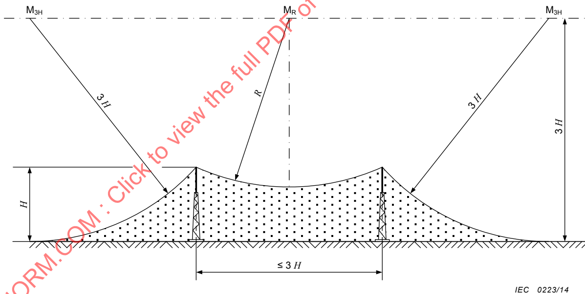
Figure E.4 – Deux paratonnerres
