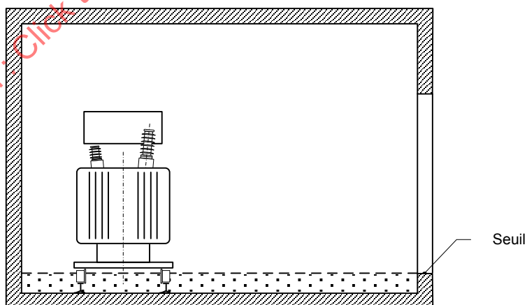
Figure 10 – Fosse avec réservoir de récupération commun intégré
