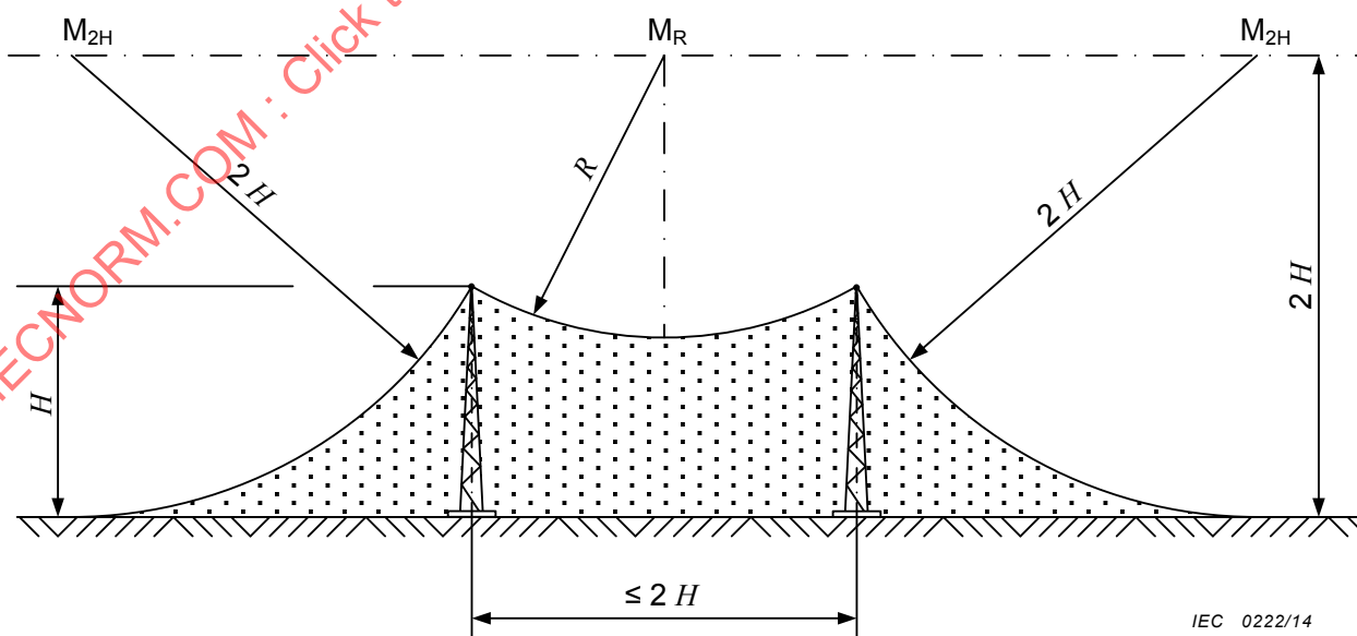
Figure E.2 – Deux câbles de garde simple
