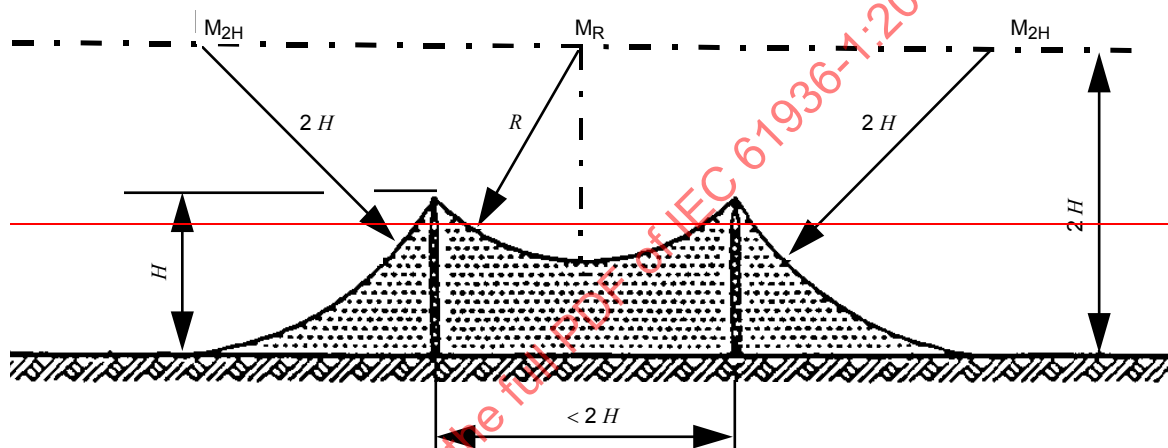
Figure E.1 – Câble de garde simple
