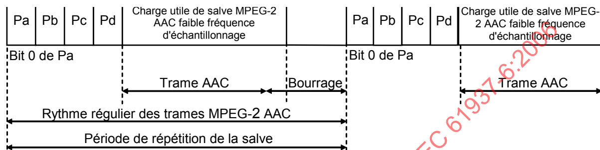
Figure 5 – Salve de données au format MPEG-2 AAC quart de rythme basse fréquence d'échantillonnage
