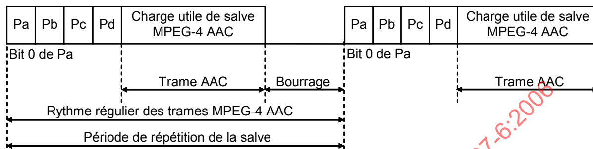
Figure 7 – Salve de données au format MPEG-4 AAC
