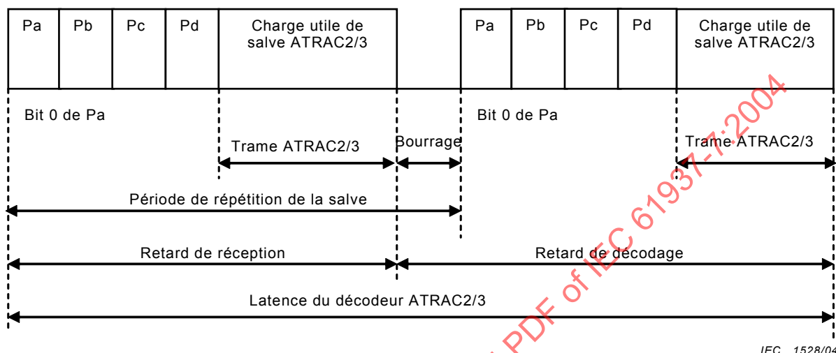
Figure 4 – Latence du décodage ATRAC2/3
