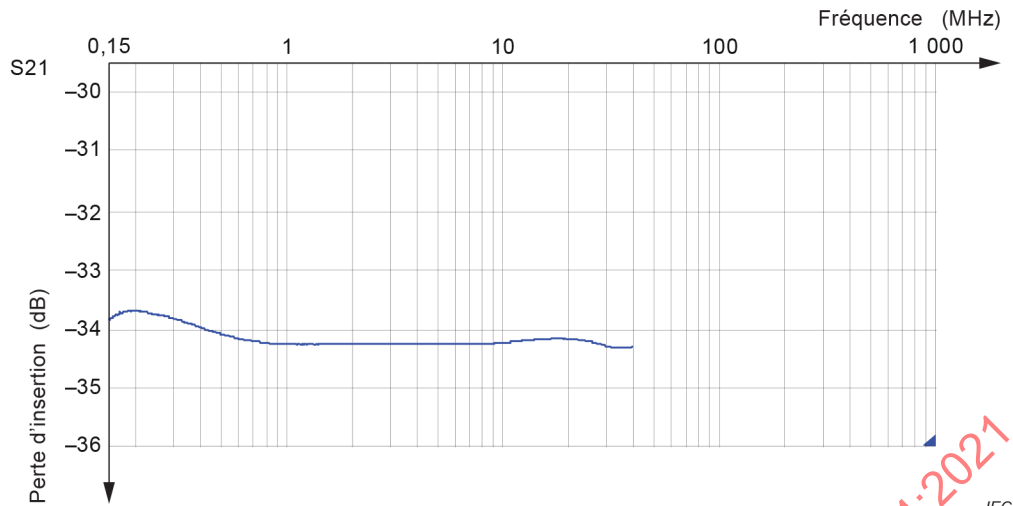
Figure A.2 – Perte d'insertion de la sonde de 1 Ω
