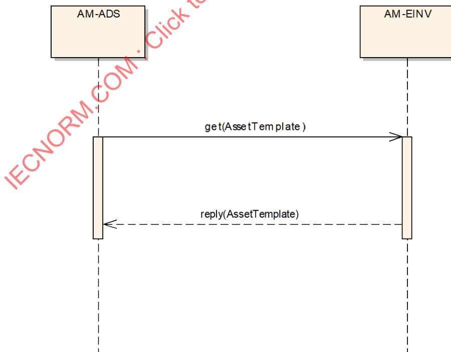
Figure 15 – Échange de requêtes AssetTemplate
