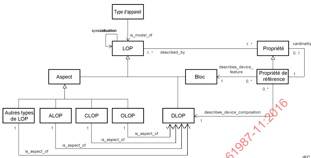
Figure 2 – Plan UML simplifié d'appareil, LOP et ses aspects
