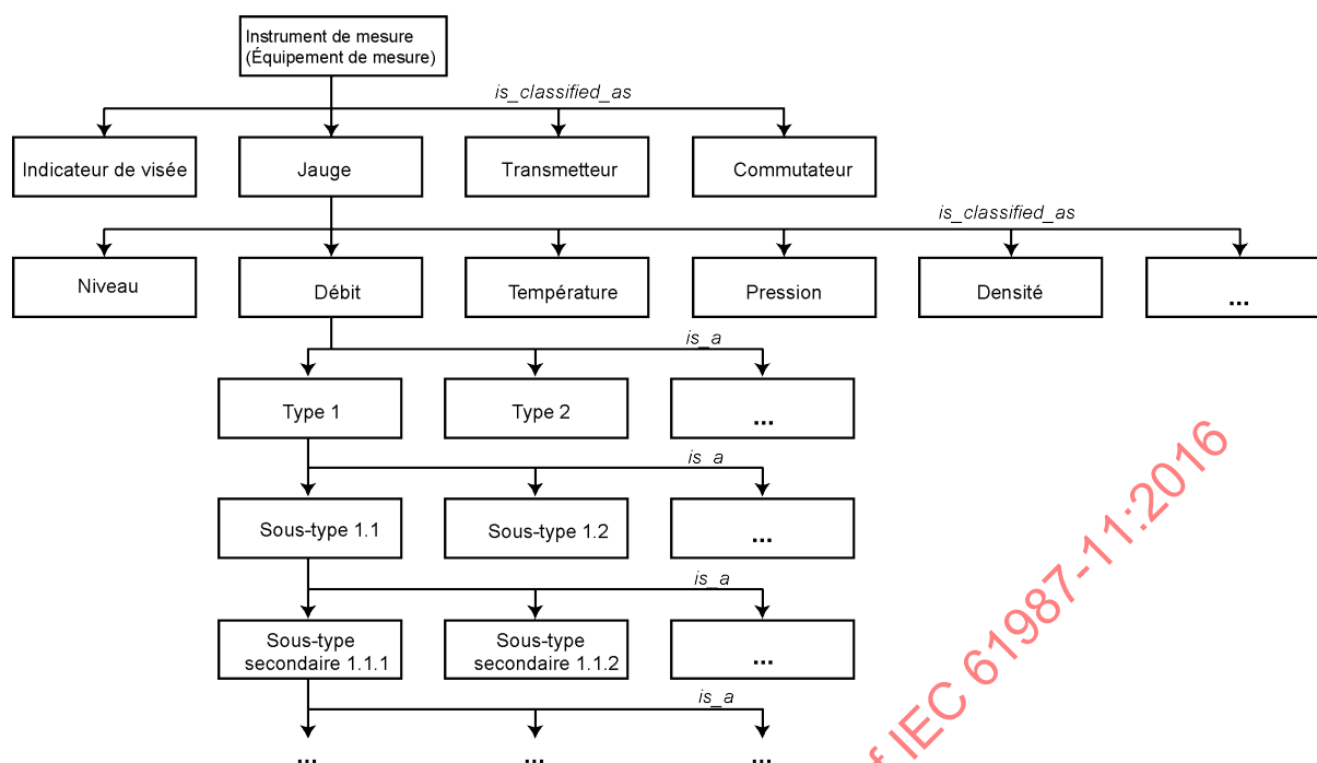
Figure 1 – Caractérisation d'un équipement de mesure
