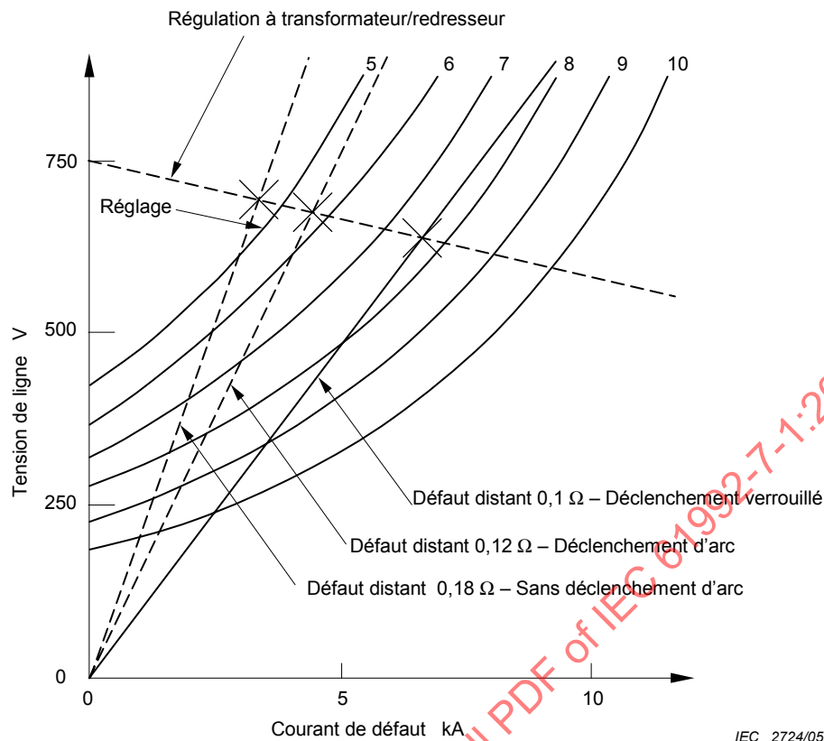
Figure 3 – Dispositif (électromagnétique) à impédance type – Caractéristiques et réglages
