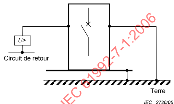
Système mis à la terre sans détection de courant
