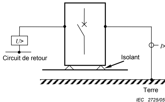
Système mis à la terre avec détection de courant
