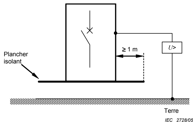
Figure 4c – Système à haute impédance
