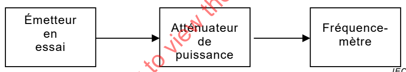
Figure 4 – Montage de mesure de l'erreur de fréquence
