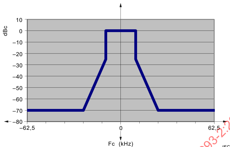
Figure 6 – Masque d'émission pour la transmission crânelée
