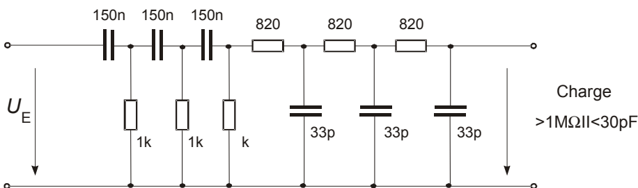
Figure 97 – Passe-bande 10 kHz à 500 kHz
