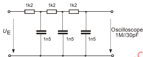
Figure 66 – Filtre A (filtre passe-bas 0 Hz à 10 kHz)
