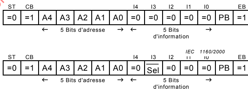
Figure 22 – Structure de la requête Delete_Address (supérieur: mode d'adressage normalisé; inférieur: mode d'adressage étendu)
