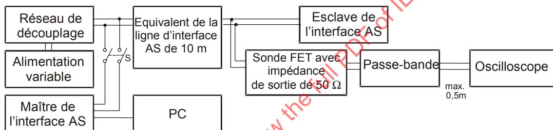
Figure 80 – Circuit d'essai
