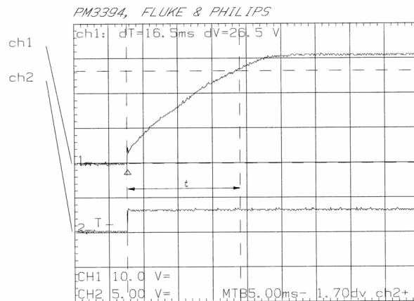
Figure 108 – Oscillogramme de consommation de courant (exemple)
