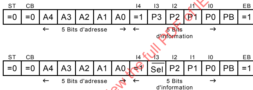
Figure 14 – Structure de la requête Write_Parameter (supérieur: mode d'adressage normalisé; inférieur: mode d'adressage étendu)
