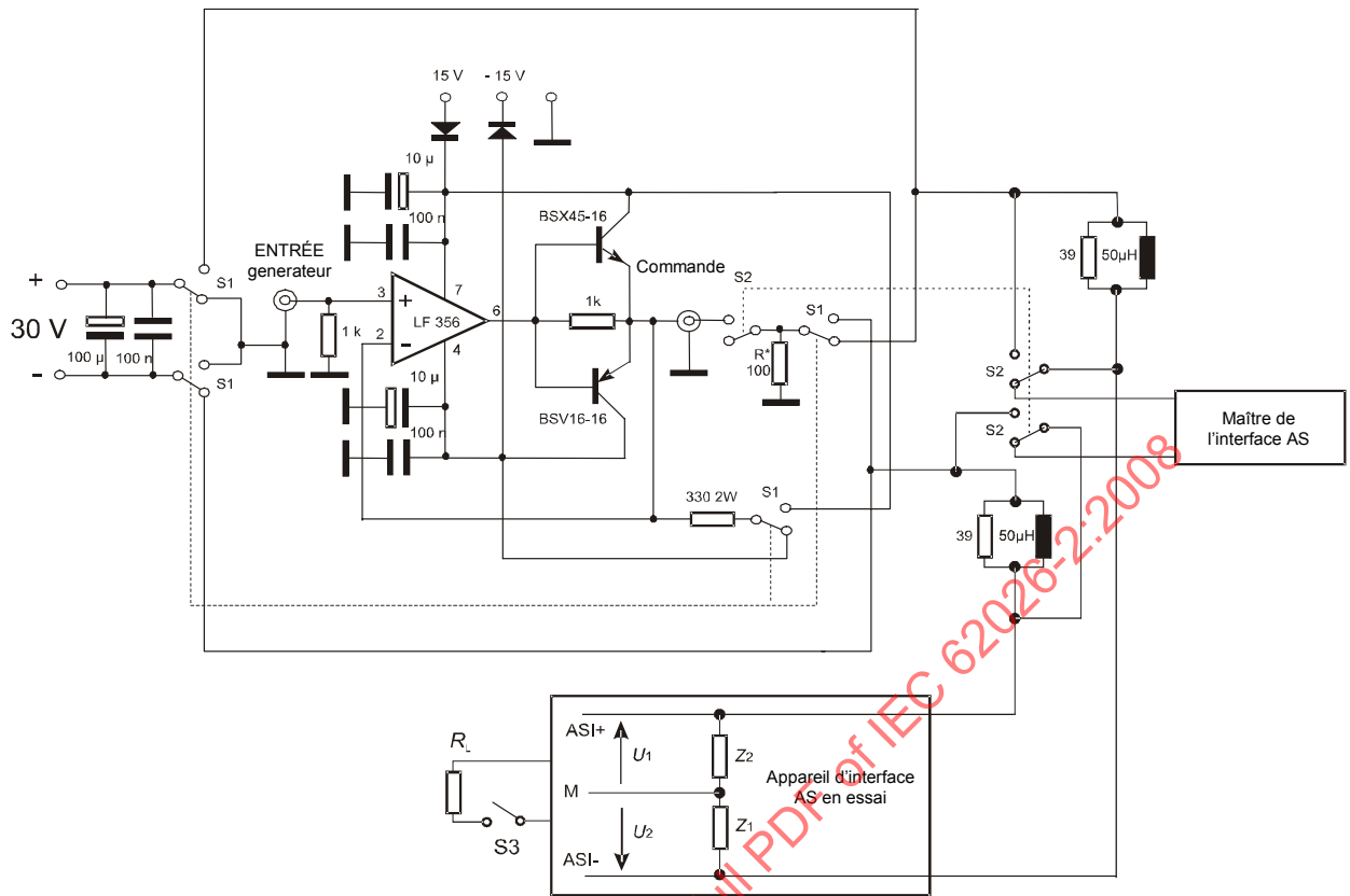
Figure 87 – Circuit d'essai
