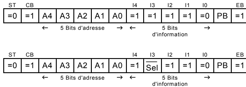
Figure 30 – Structure de la requête Read_Status (supérieur: mode d'adressage normalisé; inférieur: mode d'adressage étendu)
