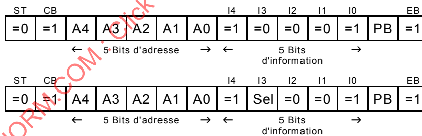
Figure 26 – Structure de la requête Read_Identification_Code (supérieur: mode d'adressage normalisé; inférieur: mode d'adressage étendu)
