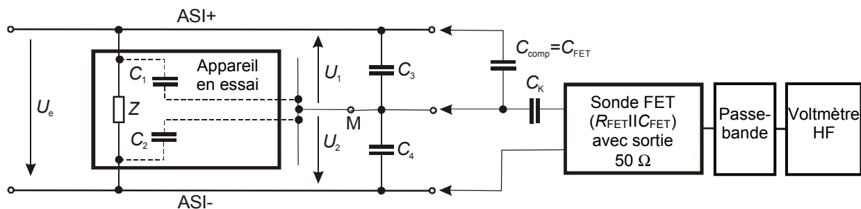
Figure 89 – Circuit d'essai (détail 2)
