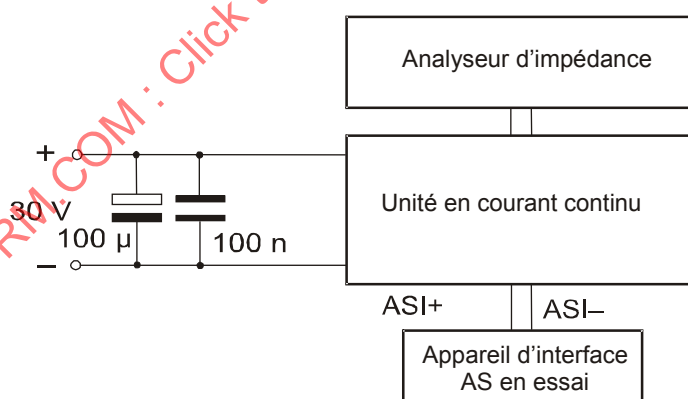
Figure 69a – Analyseur d'impédance
