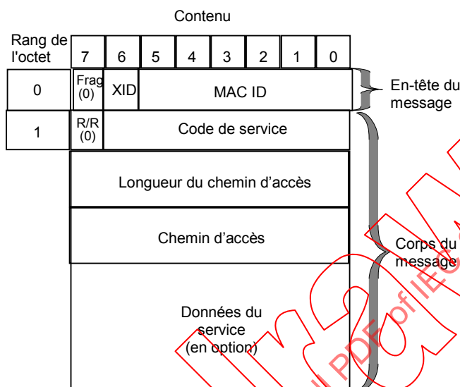
Figure 13 – Format d'un message de requête explicite non fragmenté, valeur 4
