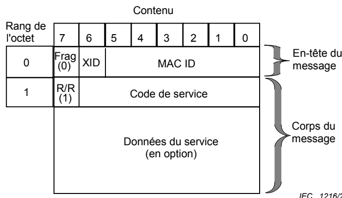
Figure 14 – Format d'un message réponse positif non fragmenté
