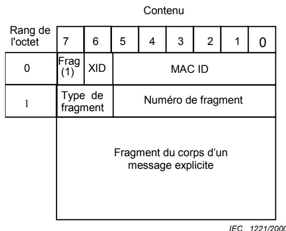
Figure 19 – Format d'un fragment de message explicite
