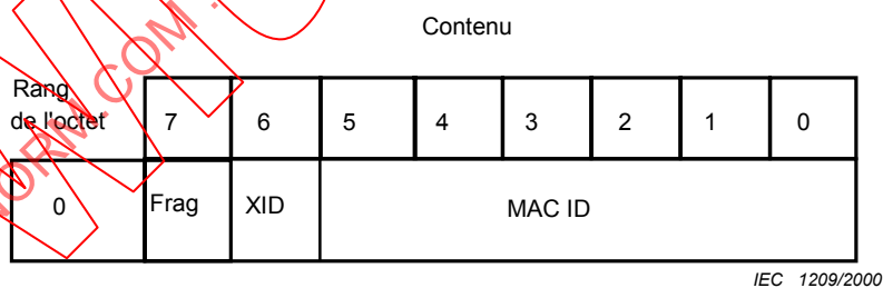
Figure 6 – Format de l'en-tête d'un message explicite
