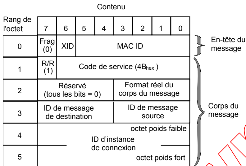
Figure 9 – Format de la réponse d'ouverture de connexion de messagerie explicite
