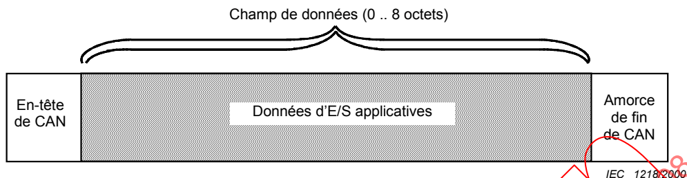
Figure 16 – Champ de données d'un message d'E/S
