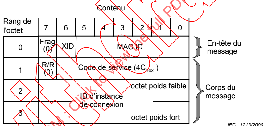
Figure 10 – Format de la requête de fermeture de connexion
