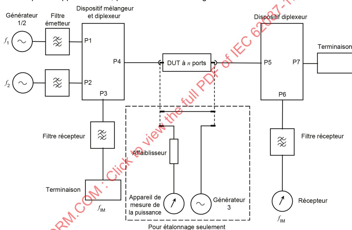
Figure 2 – Montage 2: Montage d'essai de l'intermodulation directe
