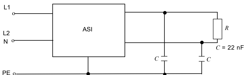
Figure 102 – Circuit d'essai pour variation du potentiel de référence induite par la charge – Sortie monophasée
