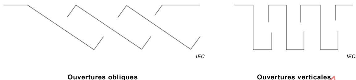
Figure 101 – Exemples de conceptions d'ouvertures destinée à empêcher l'accès vertical
