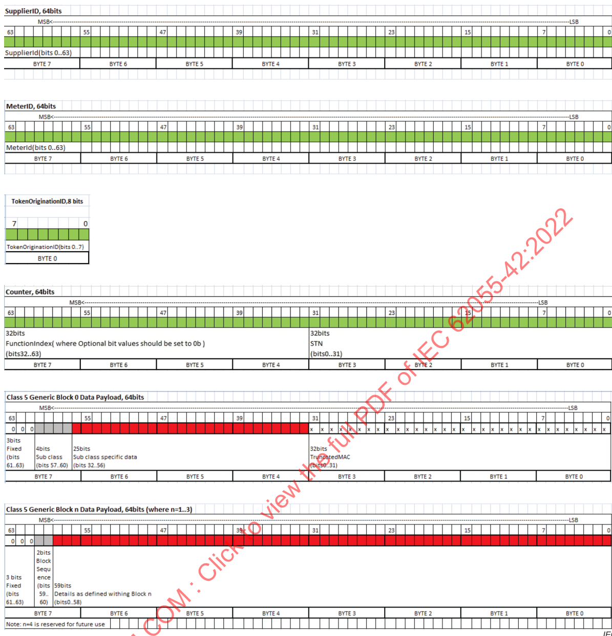
Figure 6 – Eléments de données génériques pour la construction de la charge utile de l'AAD pour la SuperTokenPayload
