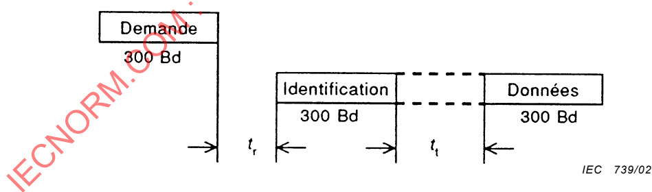
Figure 13 – Protocole d'émission en mode de protocole C pour lecture des données sans acquiescement du TSP
