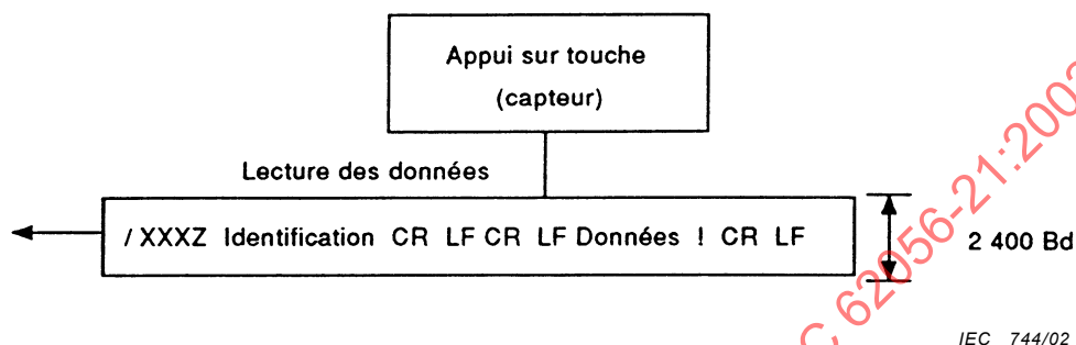
Figure 18 – Schéma du mode de protocole D
