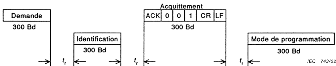
Figure 17 – Protocole d'émission en mode de protocole C. Commutation en mode de programmation avec rejet du débit proposé
