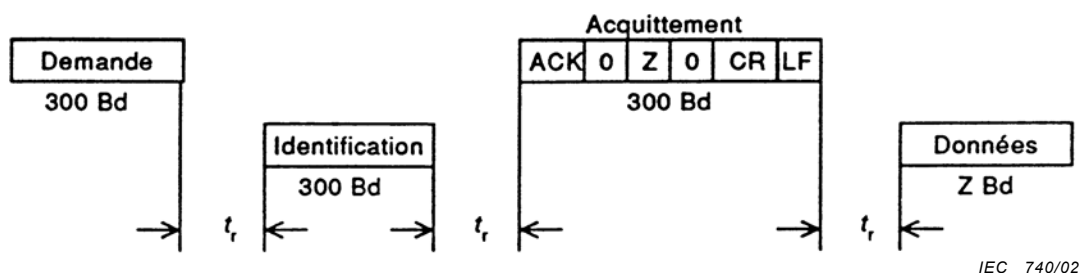
Figure 14 – Protocole d'émission en mode de protocole C avec lecture des données après confirmation du débit proposé
