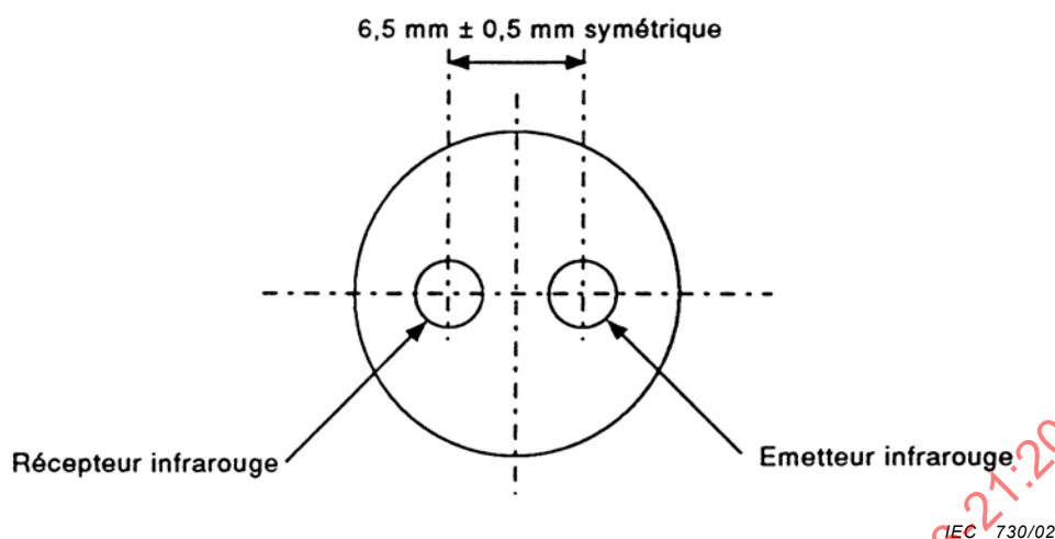
Figure 4 – Vue en direction du port optique
