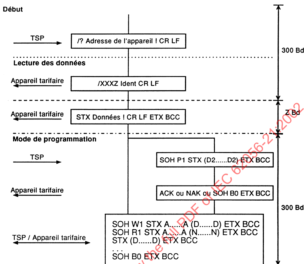
Figure 10 – Schéma du mode de protocole B
