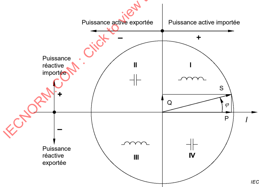
Figure 1 – Définition des quadrants pour la puissance active et réactive
