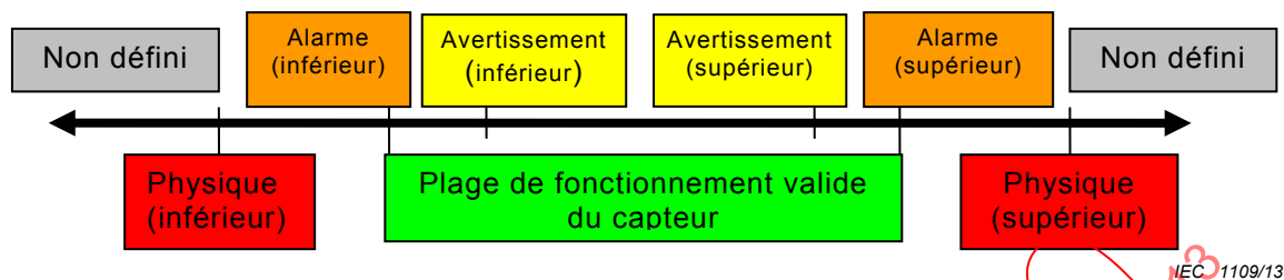
Figure 14 – Définition des seuils supérieur et inférieur
