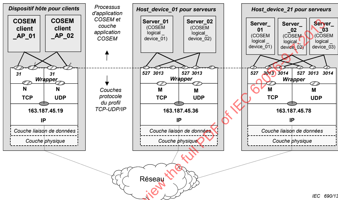
Figure 3 – Aménagement d'identification/d'adressage dans le où les profils basés sur TCP-UDP/IP
