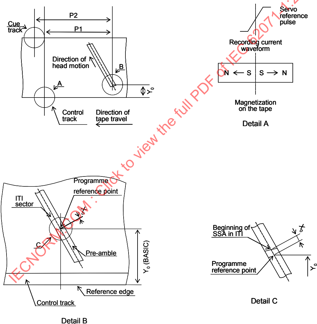
Figure 2 – Emplacements et dimensions des pistes enregistrées du format à 50 Mb/s
