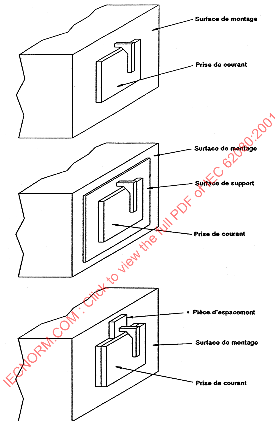
Figure 5 – Exemples de l'application du calibre de la figure 4 sur des capots fixés sans vis sur une surface de montage ou de support
