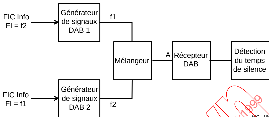
Figure 6 – Schéma fonctionnel de mesure du temps d'acquisition après la perte de synchronisation
