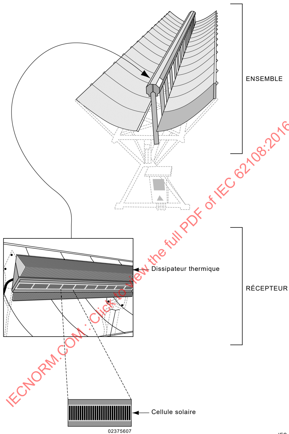
Figure 2 – Schéma d'un système PV à concentration à réceptacle avec focalisation linéaire
