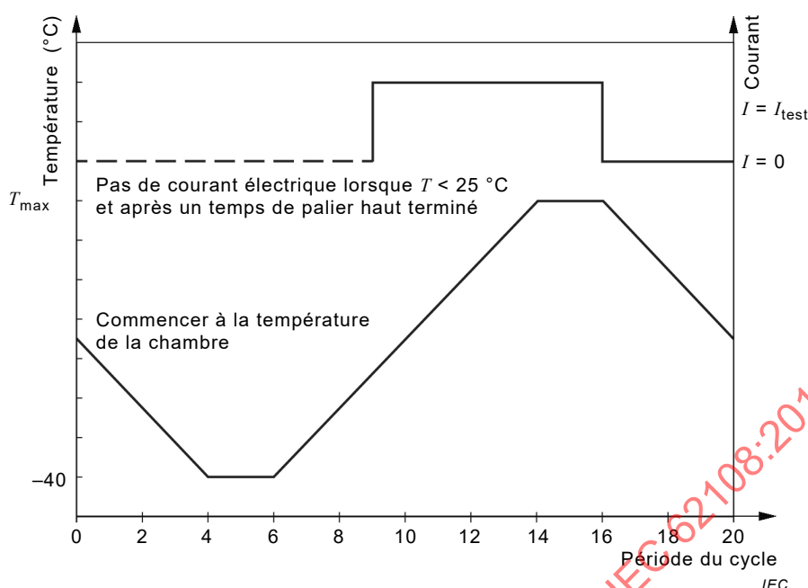
Figure 8 – Profil de température et de courant de l'essai de cyclage thermique (pas à l'échelle)
