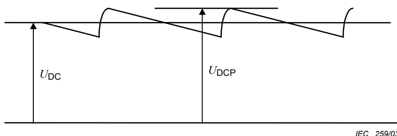
Figure 3 – Forme d'onde typique pour une tension de fonctionnement c.c.
