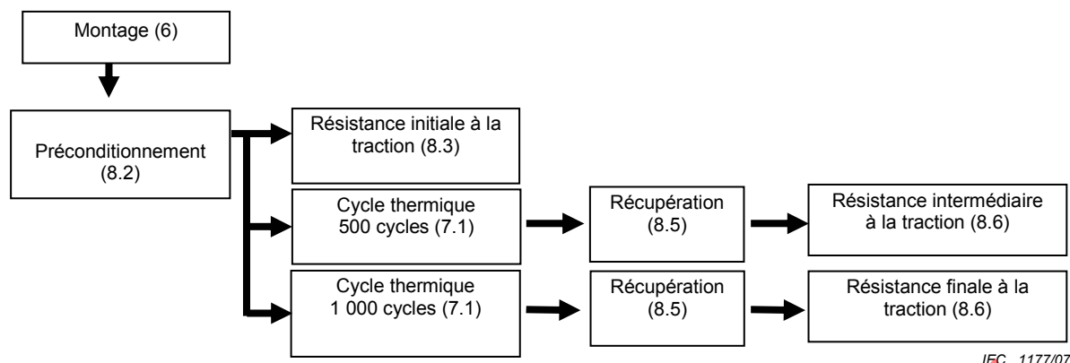
Figure 5 – Procédure d'essai
