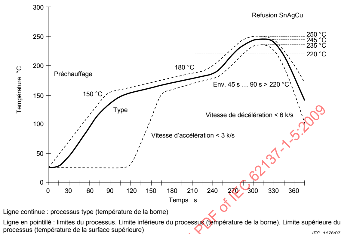
Figure 3 – Profil de température typique pris par un équipement de brasage par fusion
