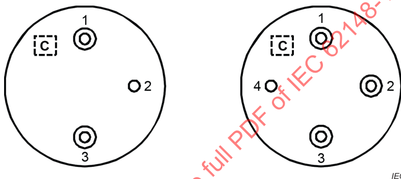
Figure 1 – Affectation de la numérotation des bornes électriques des boîtiers de type TO CAN à 3 broches et 4 broches avec code C de couleurs facultatif pour la configuration des broches
