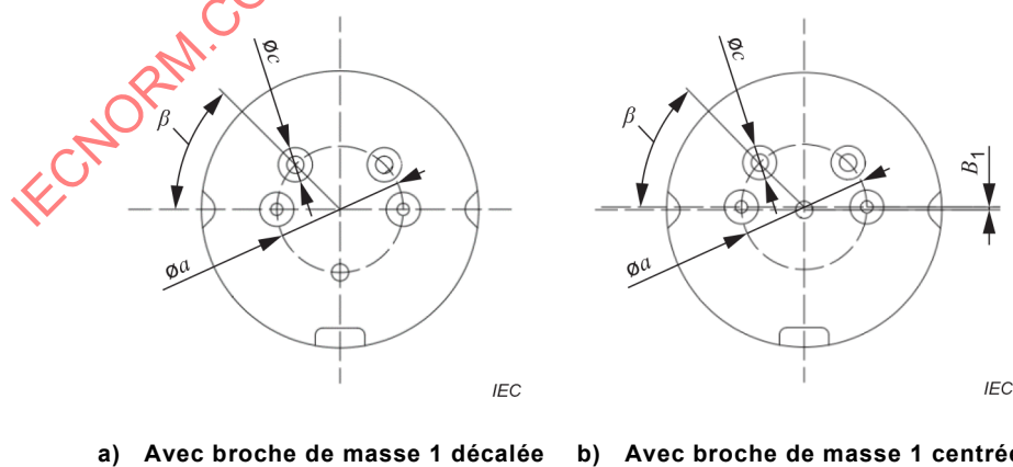
Figure 9 – Disposition des broches pour les boîtiers TO-can à 5 broches
