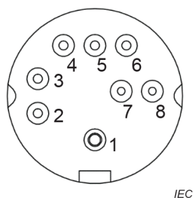
Figure 3 – Affectation de la numérotation des bornes électriques pour les boîtiers TO-can de type à 8 broches avec unité de régulation de température
