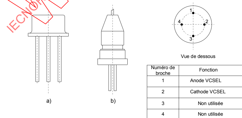
Figure A.1 – Dispositifs VCSEL TO CAN a) et à fibres amorces b) 850 nm sans photodiode de contrôle
