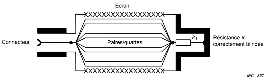
Figure 4 – Préparation de l'échantillon en essai pour les câbles symétriques
