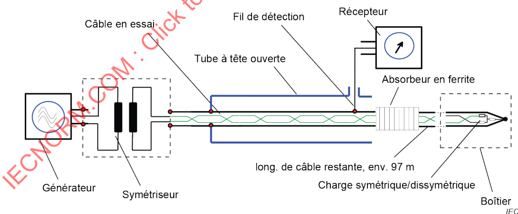
Figure 2 – Affaiblissement de couplage, principe de montage d'essai avec symétriseur et tête ouverte
