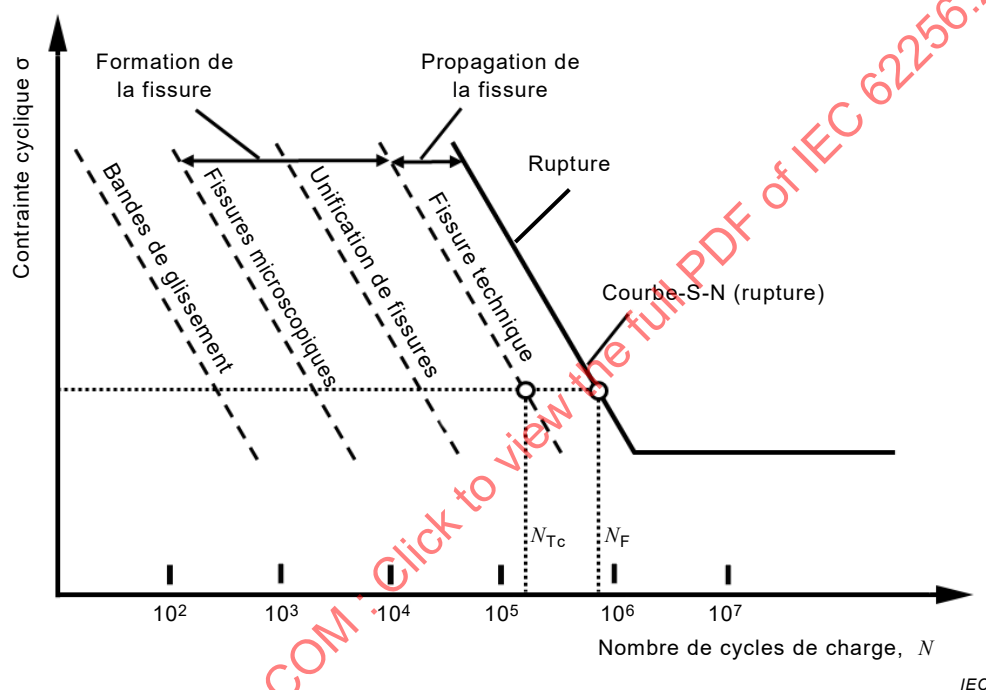
Figure 5 – Comportement schématisé aux différents stades du processus de fatigue
