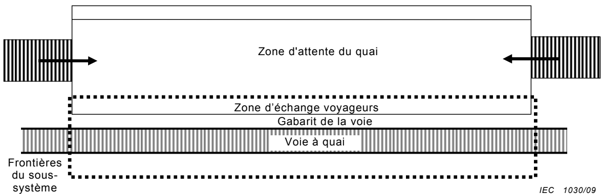
Figure 2 – Frontières du sous-système station
