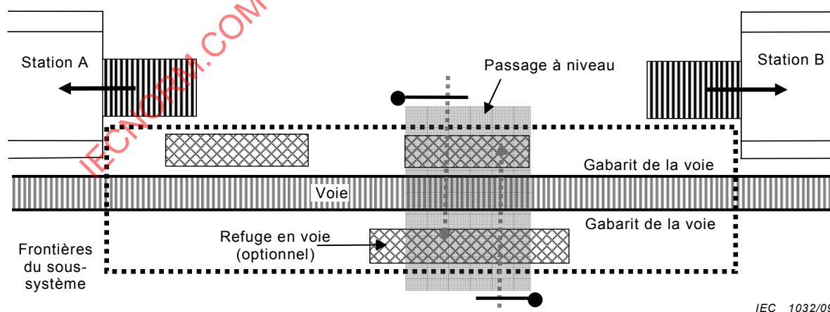
Figure 4 – Frontières du sous-système « voie entre stations » avec passage à niveau
