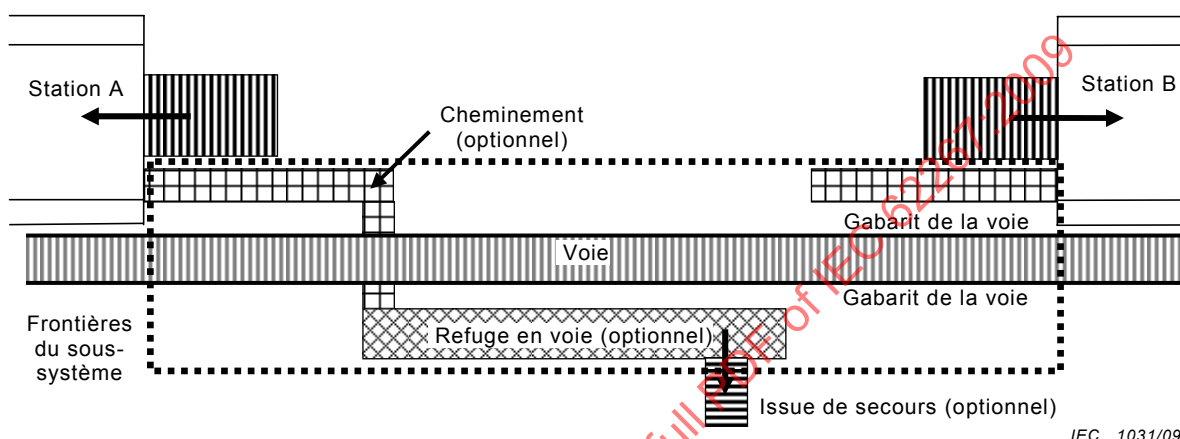
Figure 3 – Frontières du sous-système « voie entre stations »
