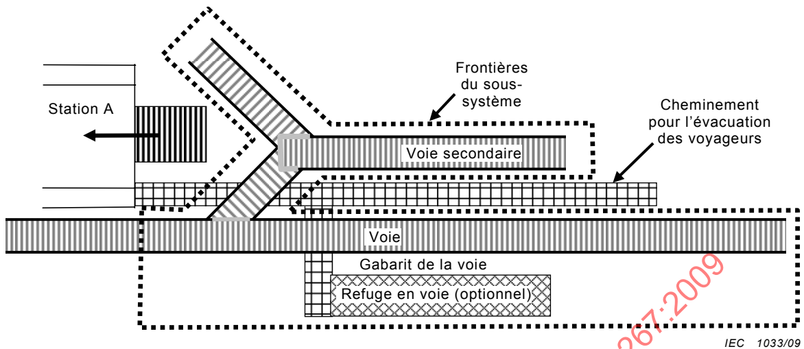
Figure 5 – Frontières du sous-système « voie entre stations » avec voies secondaires
