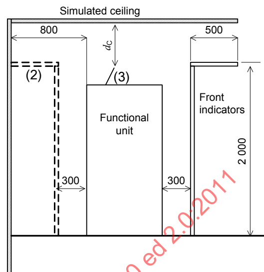
End elevation
