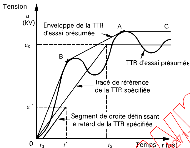
Figure 41 – Exemple d'une TTR d'essai présumée comportant une enveloppe à quatre paramètres répondant aux conditions imposées pour l'essai de type: cas de la TTR spécifiée comportant un tracé de référence à deux paramètres
