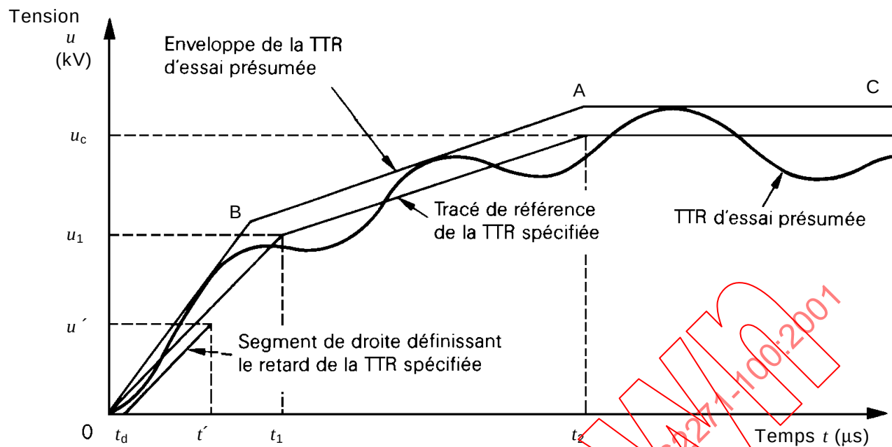
Figure 39 – Exemple d'une TTR d'essai présumées comportant une enveloppe à quatre paramètres et répondant aux conditions imposées pour l'essai de type: cas de la TTR spécifiée comportant un tracé de référence à quatre paramètres
