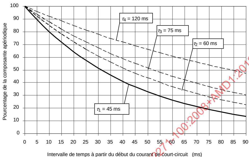
Figure 9 – Pourcentage de la composante apériodique en fonction de l'intervalle de temps à partir du début du courant de court-circuit pour les différentes constantes de temps normale \tau_1 et pour les constantes de temps \tau_2 , \tau_3 et \tau_4 des applications particulières
