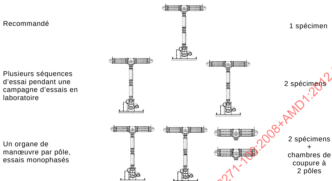
Figure 21 – Nombre permis de spécimens pour les essais d'établissement et de coupe, illustration des spécifications de 6.102.2
