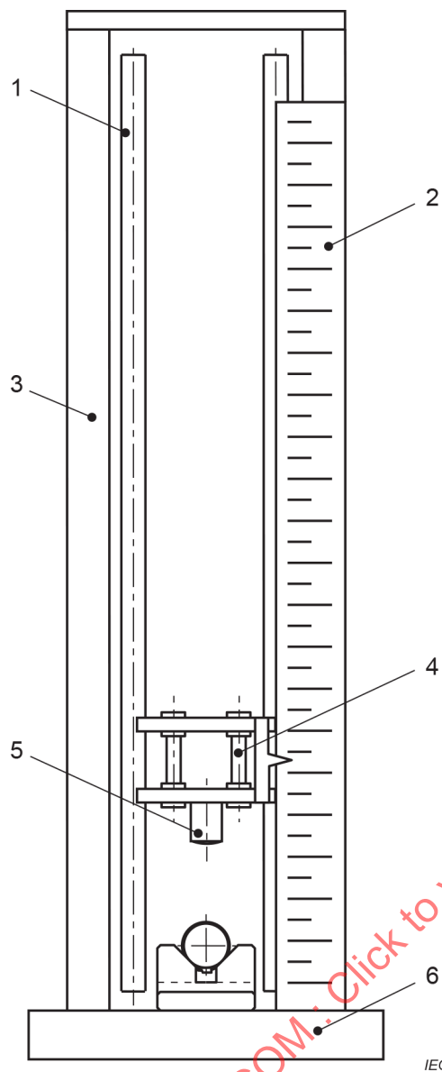
Figure 4 a) – Configuration de l'appareil d'essai
