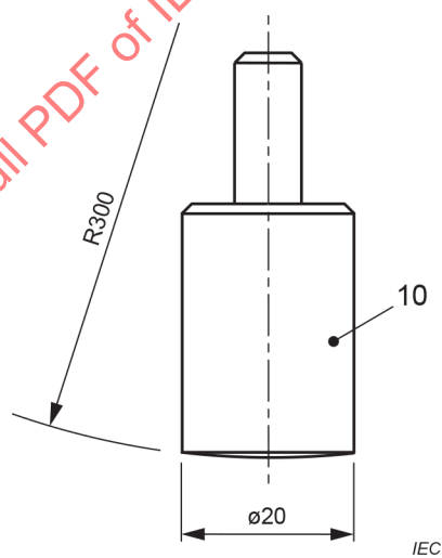
Figure 4 d) – Détails du marteau
