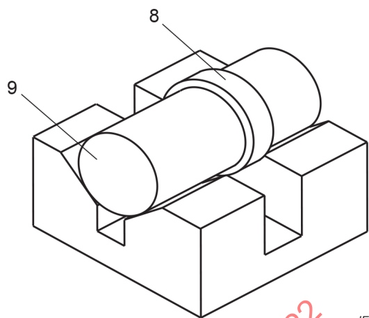
Figure 4 c) – Position de la lanière
