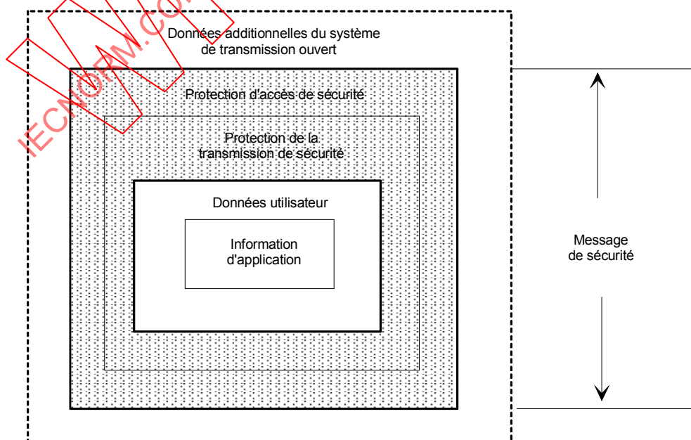
Figure 2 – Modèle d'un message de sécurité
