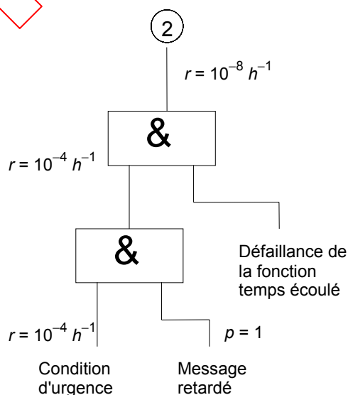
Figure C.3 – Arbre des défaillances pour le cas 2
