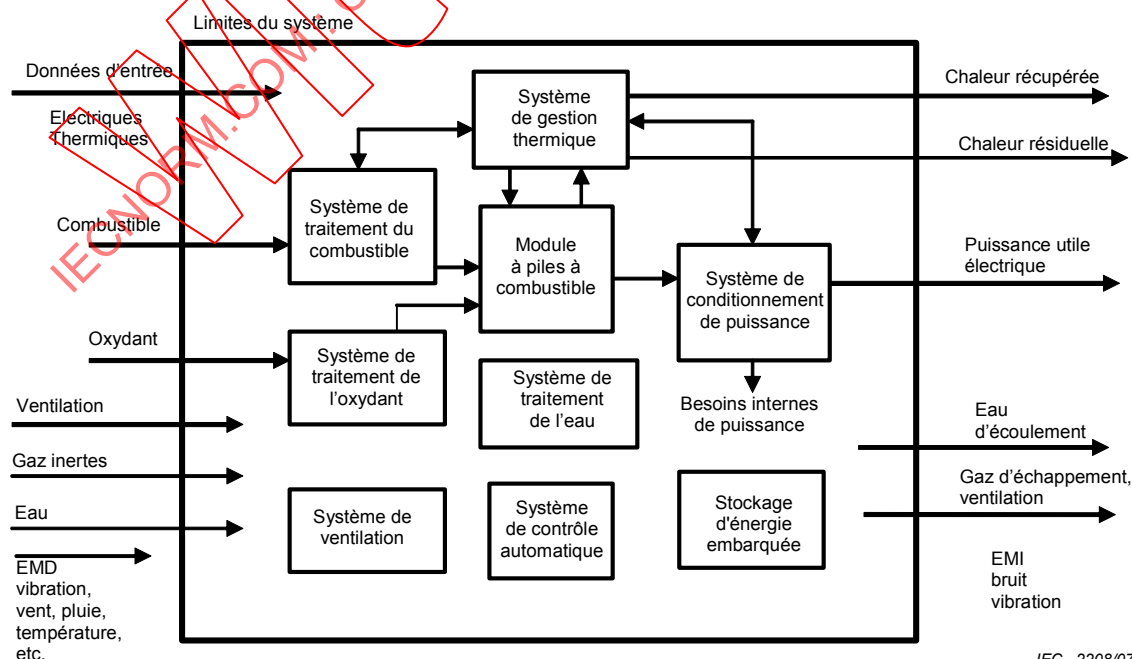
Figure 1 – Système à piles à combustible
