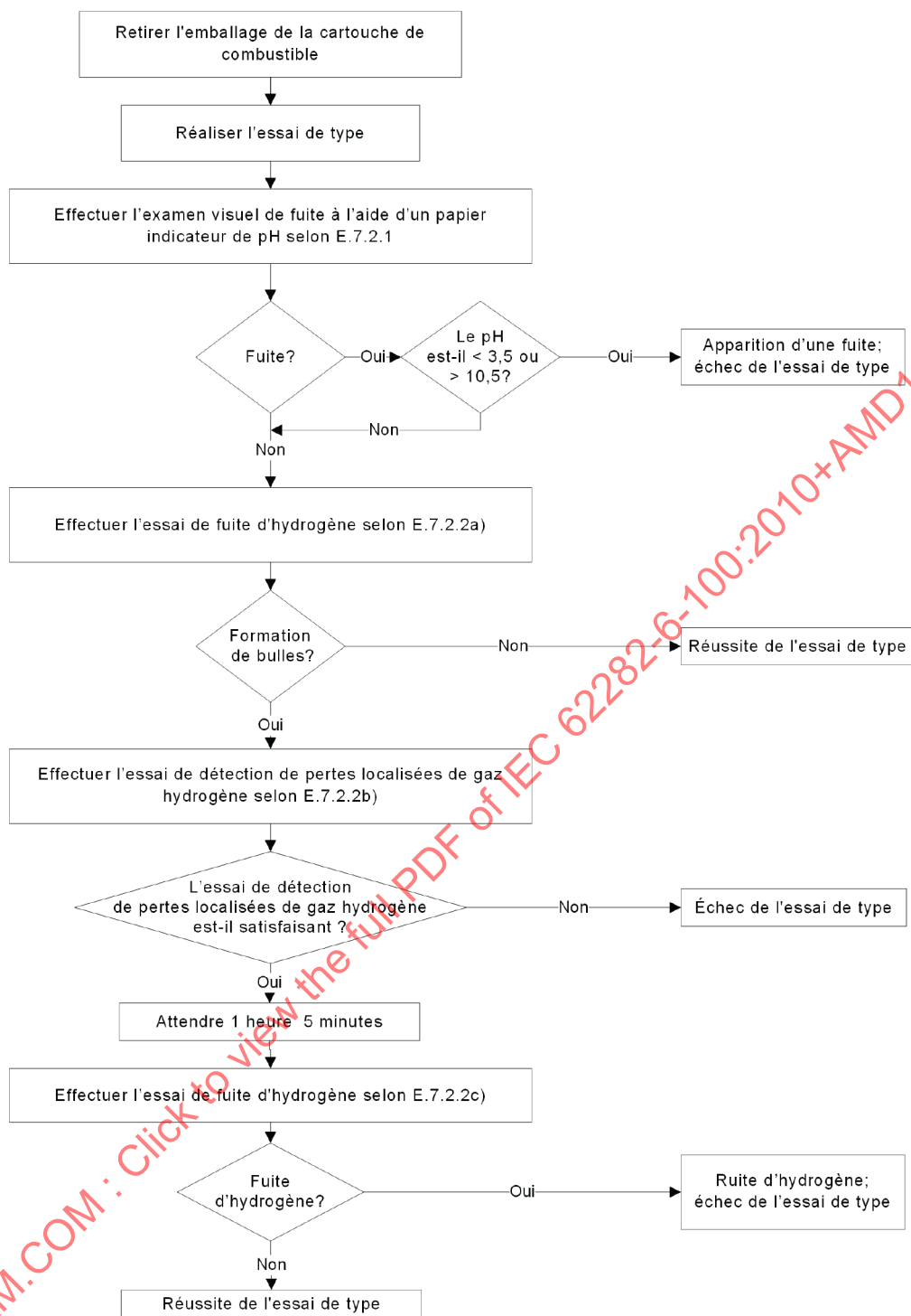
Figure E.3 – Diagramme d'essai de fuite et de perte de masse de la cartouche de combustible et de fuite d'hydrogène pour l'essai de cycles de températures et l'essai d'exposition à température élevée – Remplace la Figure 3
