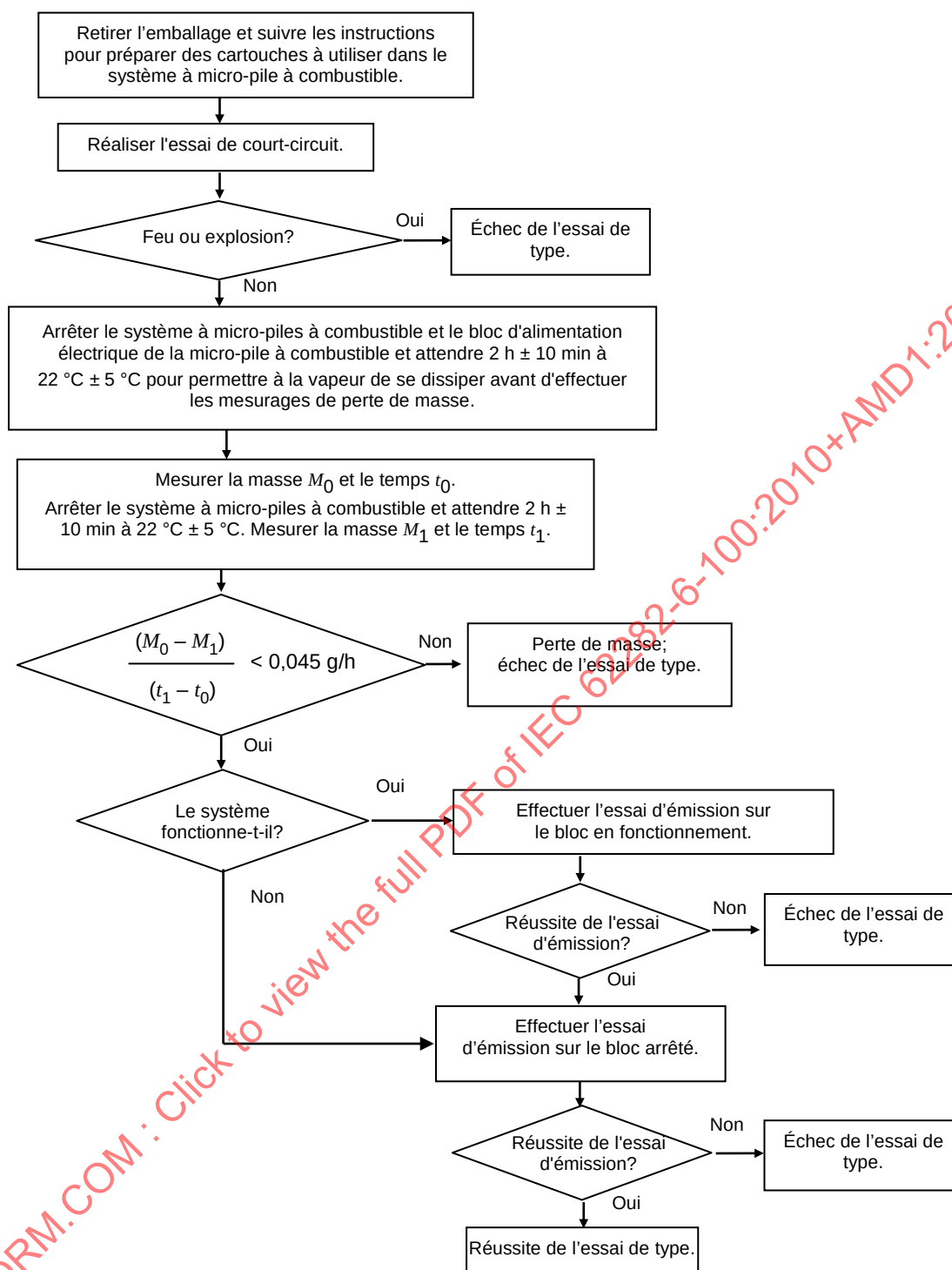
Figure H.5 – Diagramme d'essai de fuite du système à micropile à combustible ou du bloc d'alimentation électrique de la micropile à combustible, et de perte de masse pour l'essai de court-circuit externe – Remplace la Figure 5
