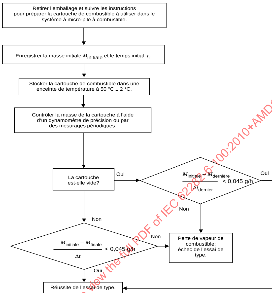
Figure H.9 – Diagramme d'essai de fuite de la cartouche de combustible et de perte de masse pour l'essai de stockage de longue durée – Remplace la Figure 9
