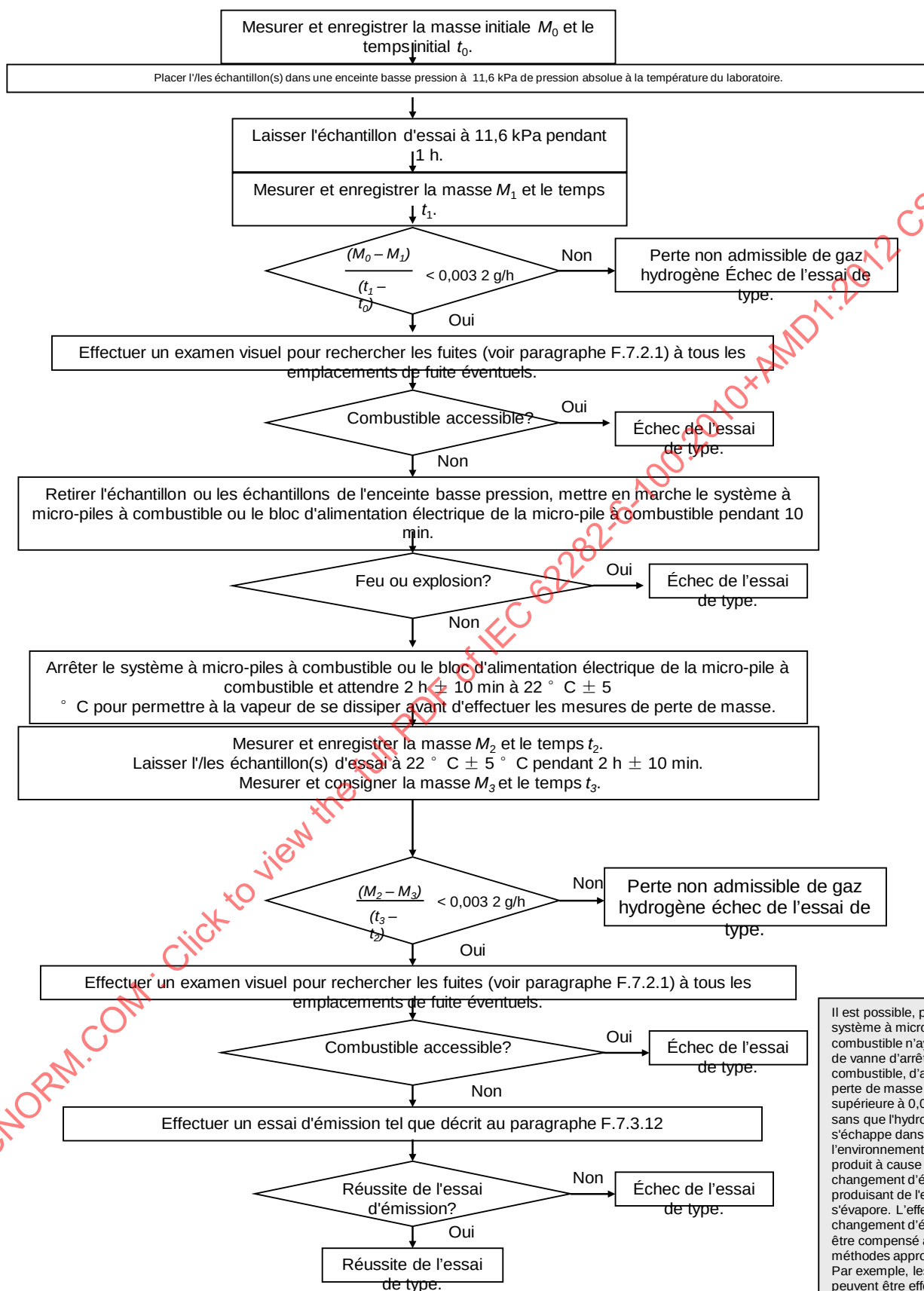
Figure F.7 – Diagramme d'essai de fuite du système à micropile à combustible ou du bloc d'alimentation électrique de la micropile à combustible, et de perte de masse gaz hydrogène pour l'essai à basse pression externe à 11,6 kPa – Remplace la Figure 7
