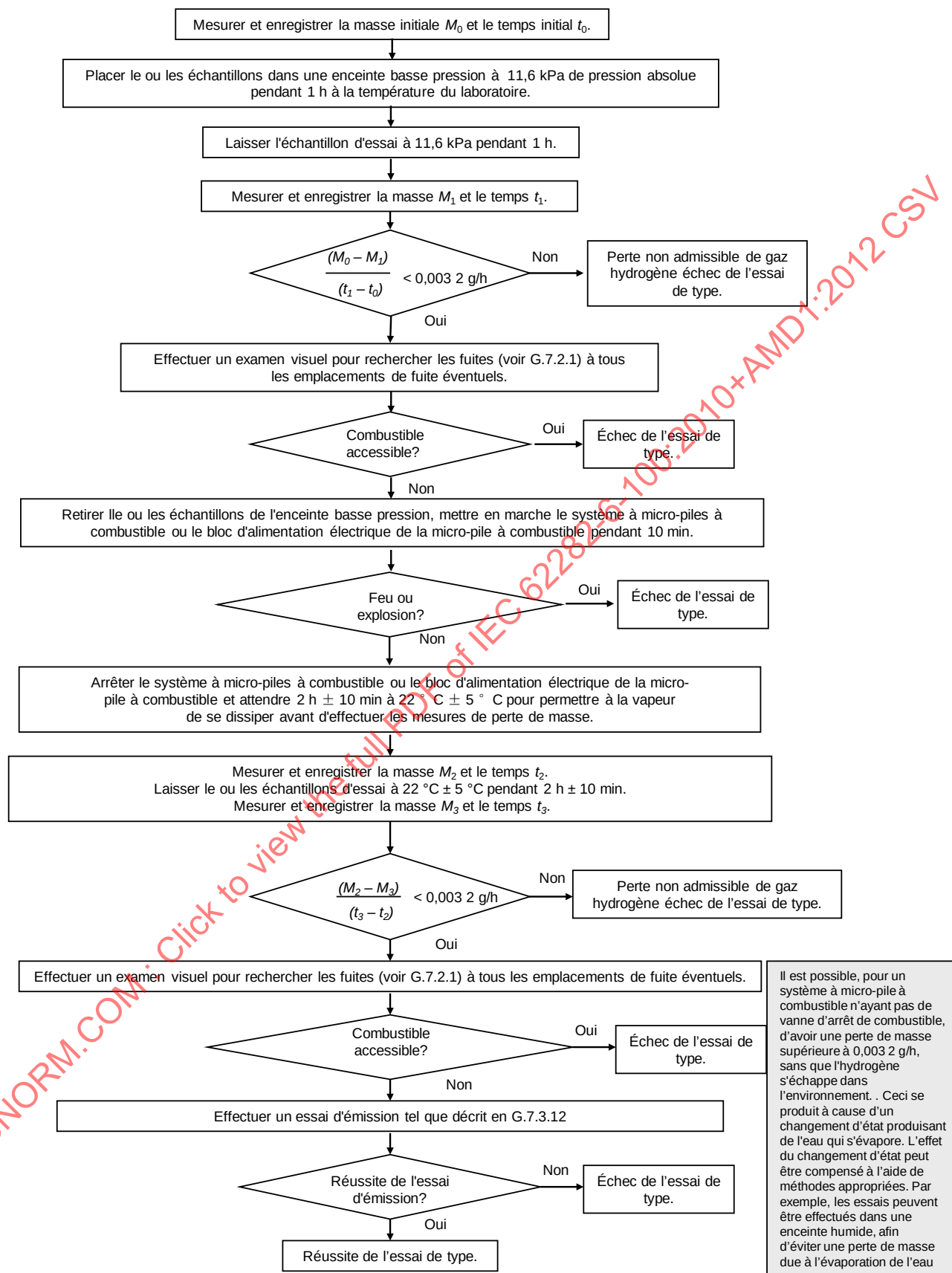
Figure G.7 – Diagramme d'essai de fuite du système à micropile à combustible ou du bloc d'alimentation électrique de la micropile à combustible, et de perte de masse pour l'essai à basse pression externe à 11,6 kPa – Remplace la Figure 7
