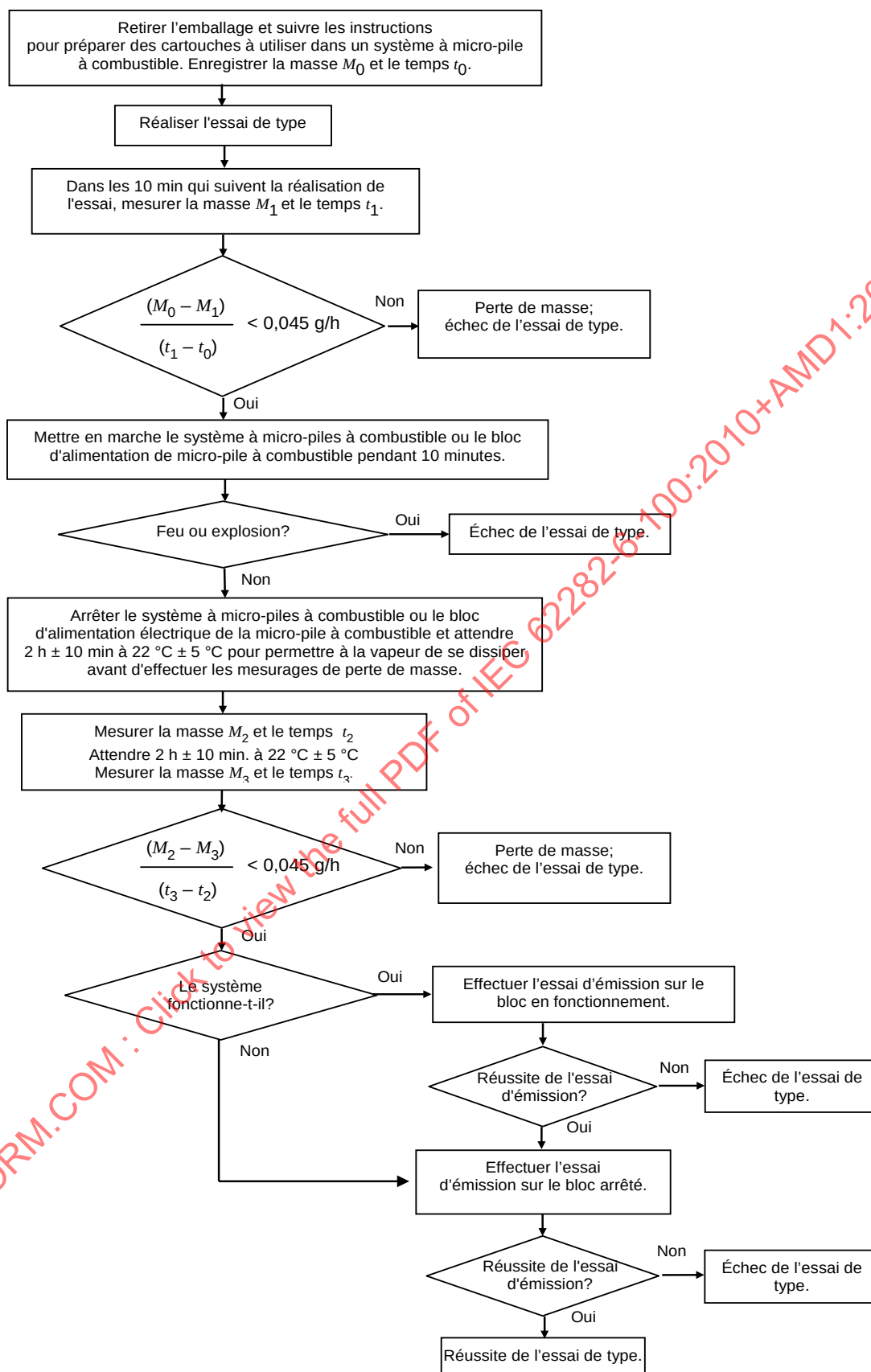
Figure H.4 – Diagramme d'essai de fuite du système à micropile à combustible ou du bloc d'alimentation électrique de la micropile à combustible, et de perte de masse pour les essais de pression différentielle, de vibrations, de cycles de températures, de chute et de charge de compression – Remplace la Figure 4
