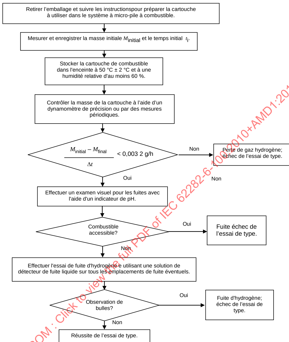
Figure G.9 – Diagramme d'essai de fuite d'hydrogène de la cartouche de combustible et de perte de masse pour l'essai de stockage de longue durée – Remplace la Figure 9
