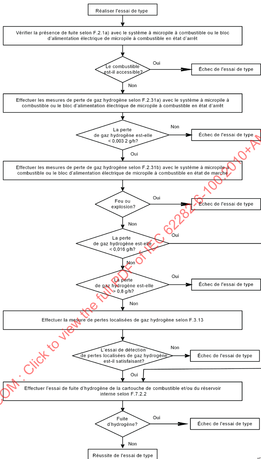
Figure F.4 – Diagramme d'essai de fuite du système à micropile à combustible ou du bloc d'alimentation électrique de la micropile à combustible et de perte de masse gaz hydrogène pour les essais de pression différentielle, de vibrations, de cycles de température, de chutes et de charge de compression – Remplace la Figure 4
