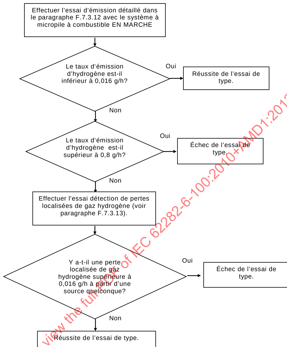
Figure F.13 – Procédure pour l'essai d'émission d'hydrogène pour le système à micropile à combustible en fonctionnement
