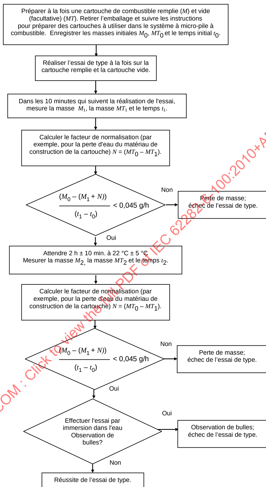
Figure H.2 – Diagramme d'essai de fuite et de perte de masse de la cartouche de combustible pour les essais de vibrations, de chute et de charge de compression – Remplace la Figure 2
