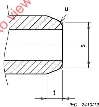
Figure 38 – Conception de la zone d'étanchéité pour le connecteur côté bloc d'alimentation électrique MFC (vue transversale)
