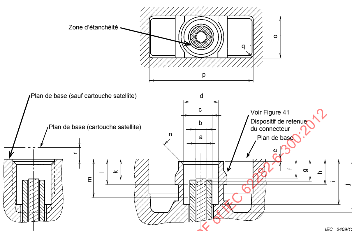
Figure 37 – Conception du connecteur côté bloc d'alimentation électrique MFC
