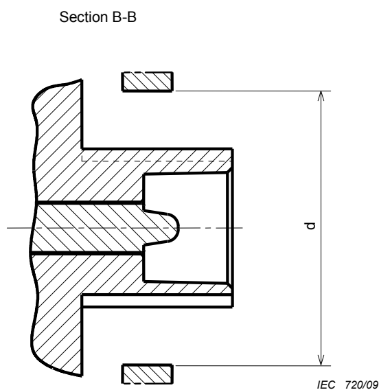
Figure 17 – Dispositif de retenue du connecteur (vue transversale avant connexion)
