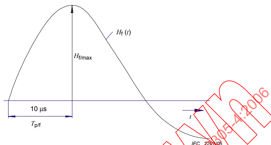
Figure A.2a – Simulation de l'élévation du champ magnétique dû à un premier choc (10/350 μs) par une seule impulsion 8/20 μs (oscillations amorties à 25 kHz)
