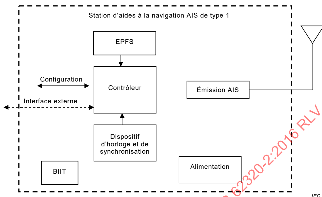
Figure 1 – Schéma de principe fonctionnel d'une station d'aides à la navigation AIS de type 1
