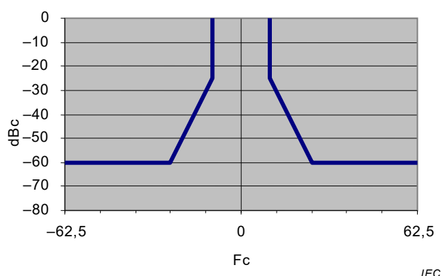
Figure 11 – Masque d'émission
