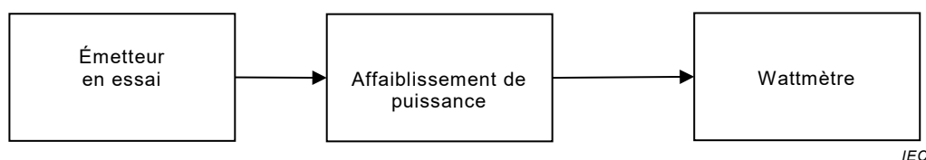
Figure 10 – Dispositif de mesure de la puissance de la porteuse
