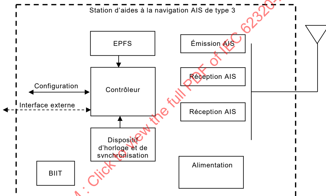
Figure 3 – Schéma de principe fonctionnel d'une station d'aides à la navigation AIS de type 3
