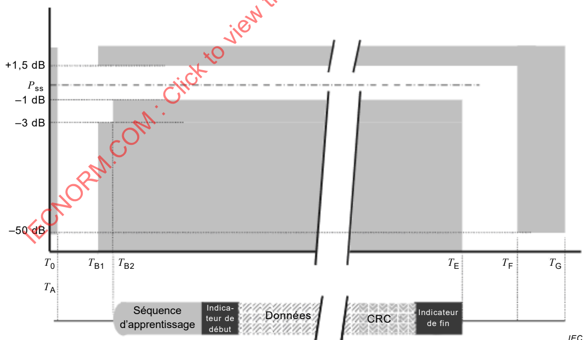
Figure 5 – Masque de la puissance en fonction du temps
