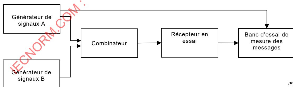
Figure 15 – Dispositif de mesure de la réjection co-canal
