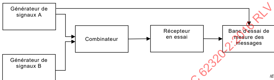
Figure 17 – Appareil de mesure PER/BER ou SINAD
