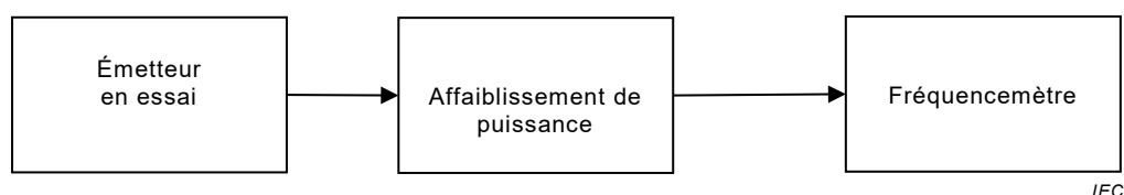
Figure 9 – Dispositif de mesure de l'erreur de fréquence
