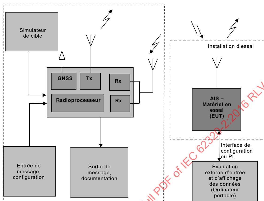
Figure 7 – Schéma de principe de configuration d'essai d'une station d'aides à la navigation AIS
