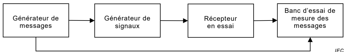
Figure 13 – Dispositif de mesure de la sensibilité
