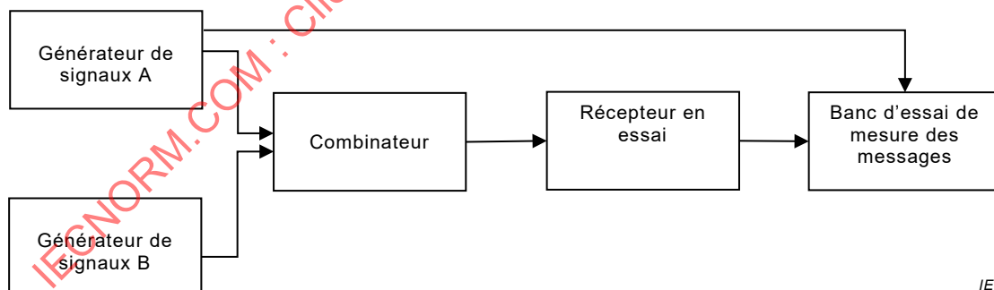
Figure 16 – Dispositif de mesure de la sélectivité pour le canal adjacent
