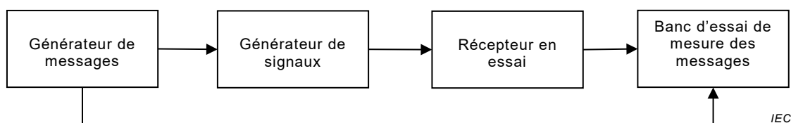
Figure 14 – Dispositif de mesure du comportement aux erreurs
