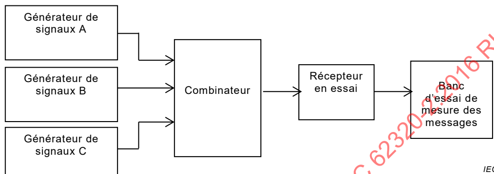
Figure 18 – Dispositif de mesure de l'intermodulation
