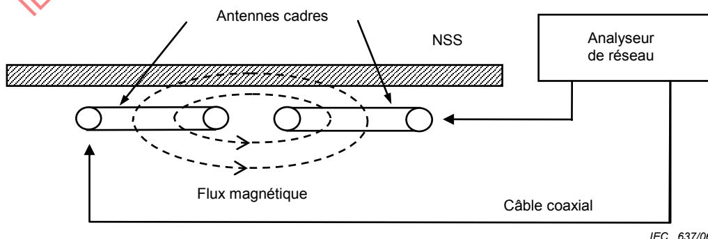
Figure 1 – Représentation schématique d'une paire d'antennes et d'une plaque réduisant le bruit
