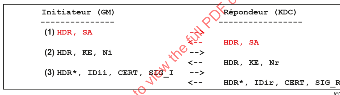
Figure 20 – Échange IKEv1 en mode principal et messages d'association de sécurité
