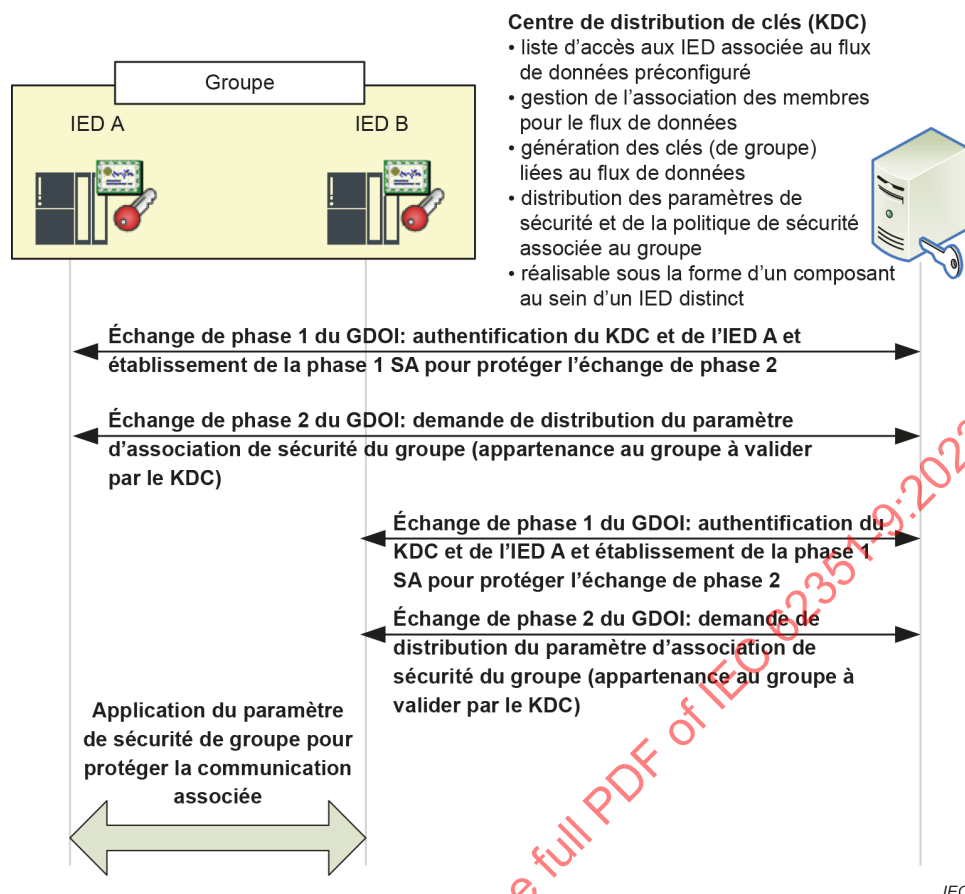
Figure 3 – Vue d'ensemble de la gestion des clés de groupe dans l'exemple de GDOI
