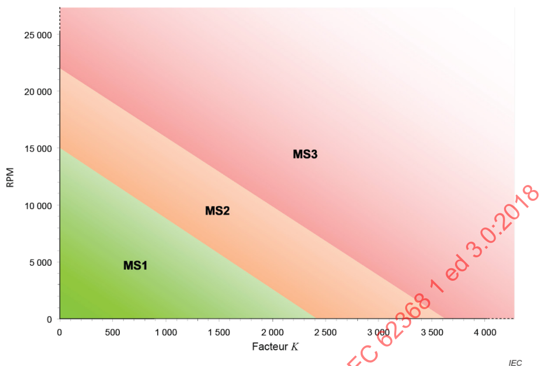
Figure 45 – Limites pour les pales mobiles de ventilateurs en matériaux autres que le plastique
