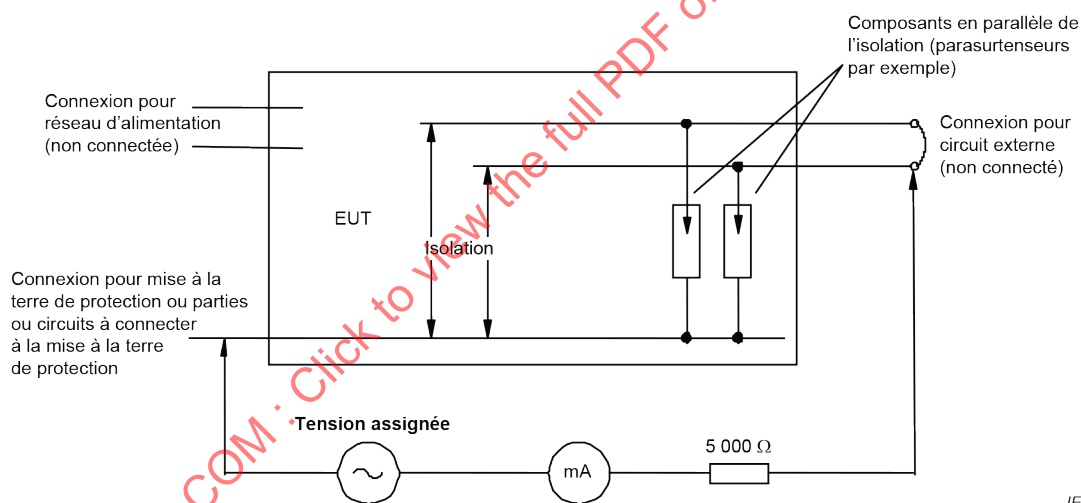
Figure 31 – Essai de séparation entre un circuit externe et la terre
