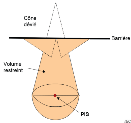
Figure 39b – Représentation d'une barrière horizontale
