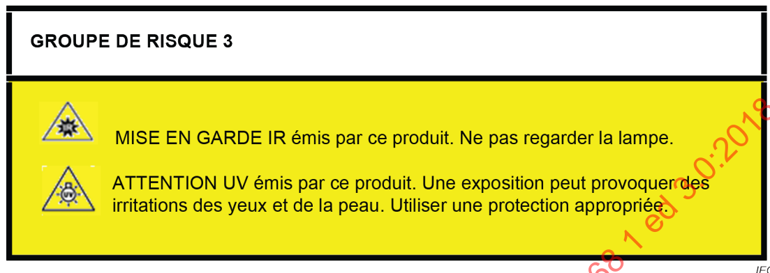
Figure 50 – Exemple d'étiquette de mise en garde pour une lampe avec plusieurs zones dangereuses du spectre
