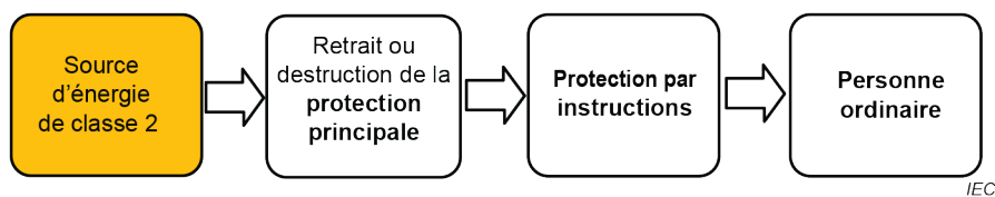
Figure 11 – Modèle pour protéger une personne ordinaire contre une source d'énergie de classe 2 dans les conditions d'entretien par une personne ordinaire
