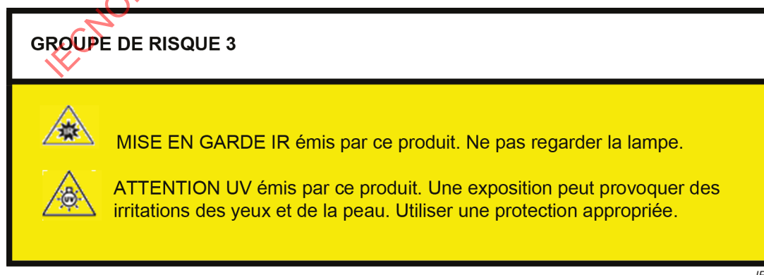
Figure 52 – Exemple d'étiquette de mise en garde pour une lampe avec plusieurs zones dangereuses du spectre
