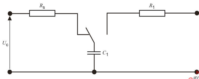
Figure D.2 – Circuit du générateur d'essai pour l'interface d'antenne
