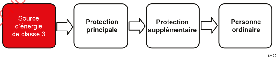
Figure 12 – Modèle de protection d'une personne ordinaire contre une source d'énergie de classe 3
