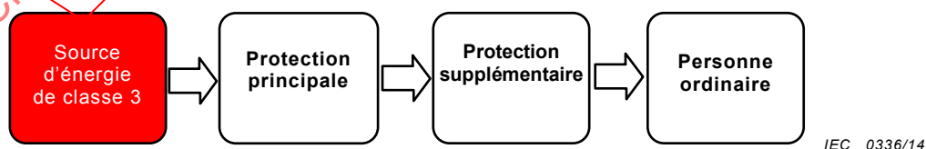
Figure 12 – Modèle pour protéger une personne ordinaire contre une source d'énergie de classe 3
