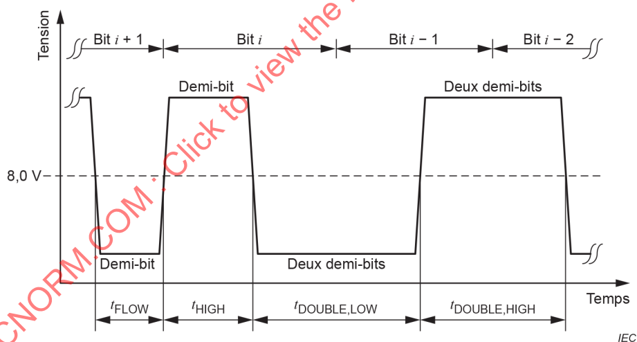
Figure 12 – Exemple de cadencement de bits
