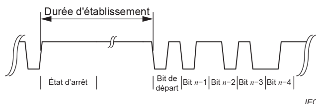
Figure 13 – Représentation de la durée d'établissement
