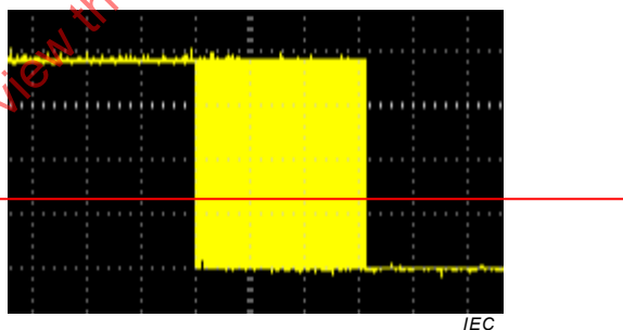
Figure 9 — Modification de l'intensité lumineuse de MAX LEVEL à la mise hors tension pour un gradateur à modulation de largeur d'impulsion
