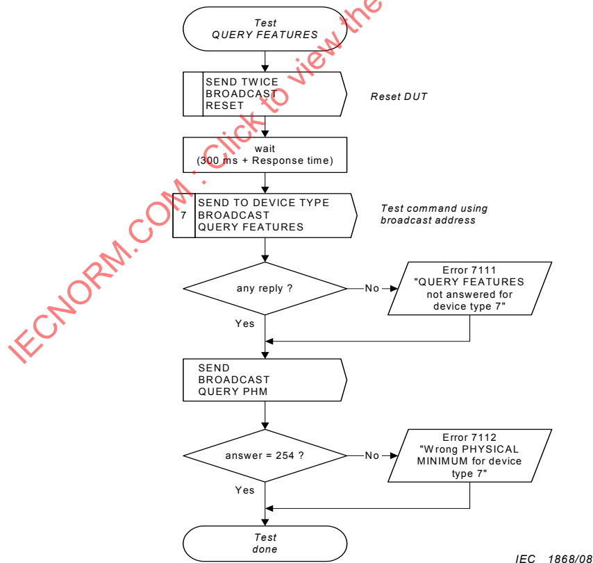
Figure 3 – Séquence d'essais QUERY FEATURES
