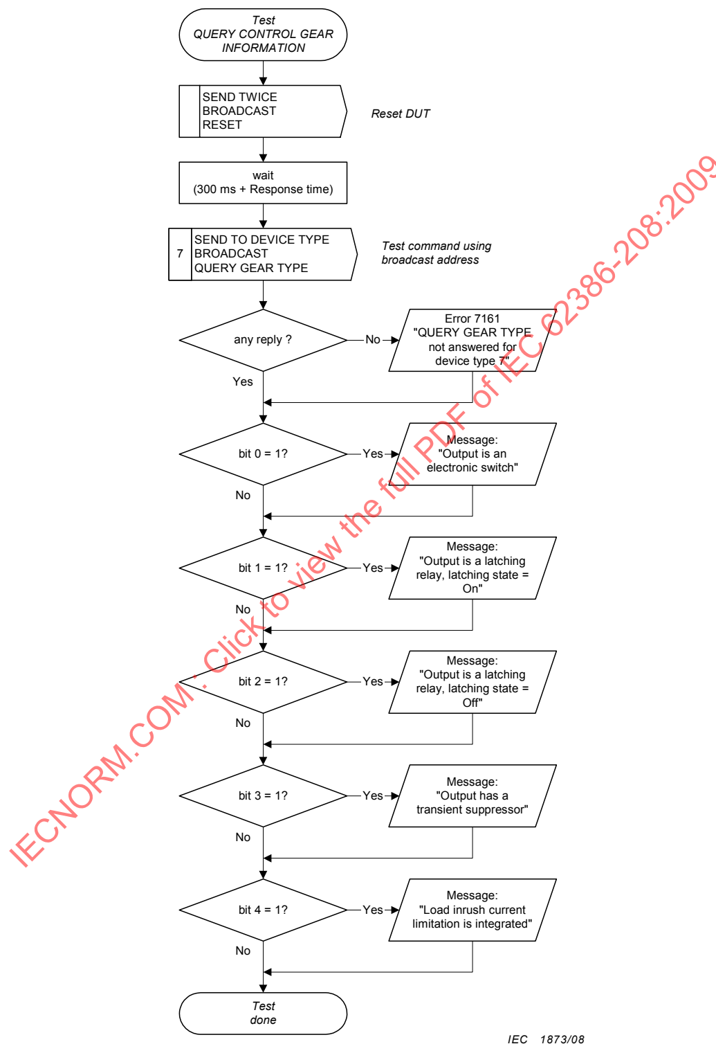
Figure 8 – Séquence d'essais QUERY Control Gear Information
