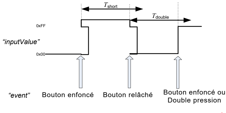
Figure 4 – Événement de double pression
